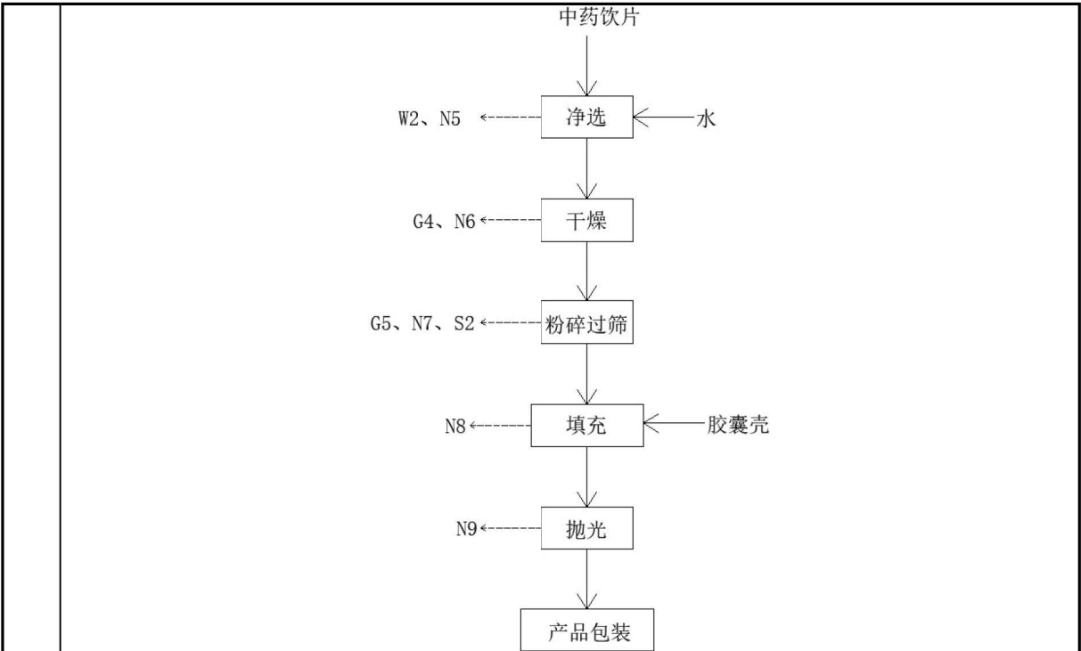
图 2-3 胶囊剂生产工艺流程图
