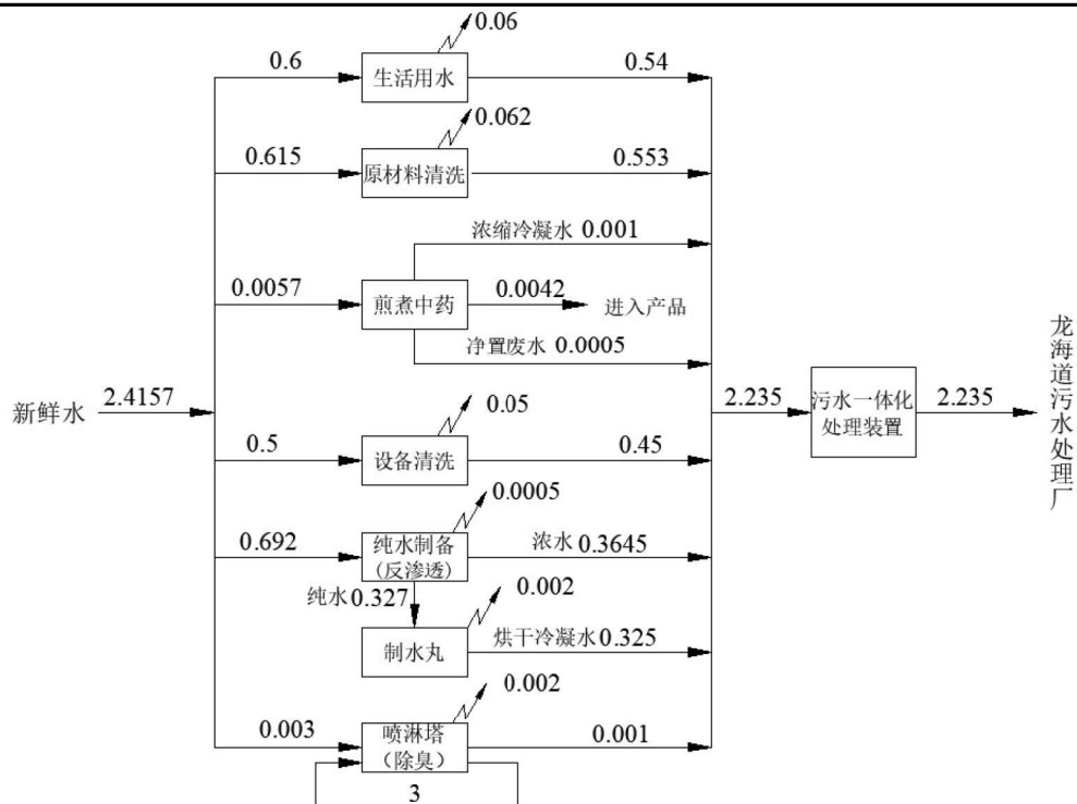
图 2-1 水平衡图 ( \text{m}^3/\text{d} )
