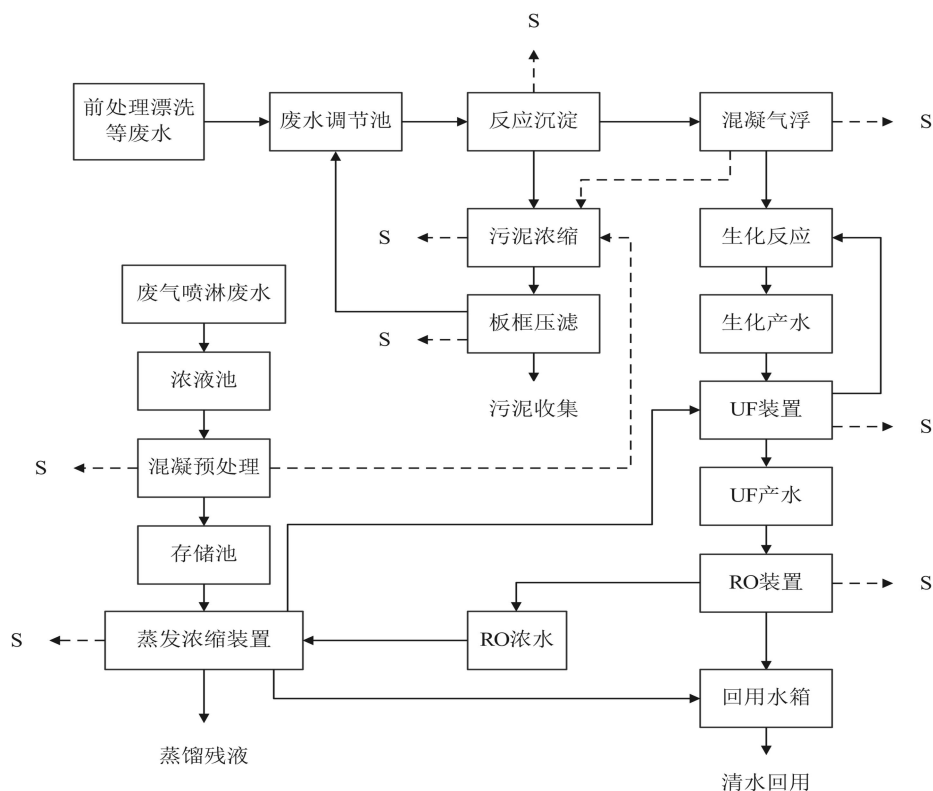
图 2-9 涂装车间废水处理工艺流程及产污节点图
