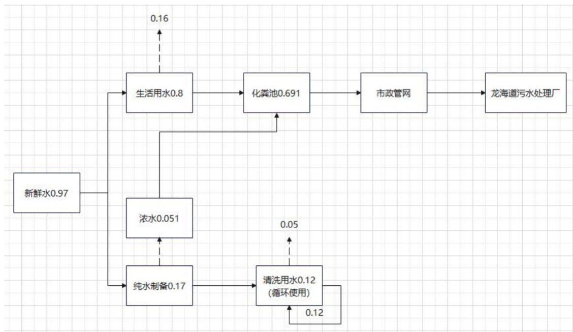
图 2-1 建设项目水量平衡图 ( \text{m}^3/\text{d} )
